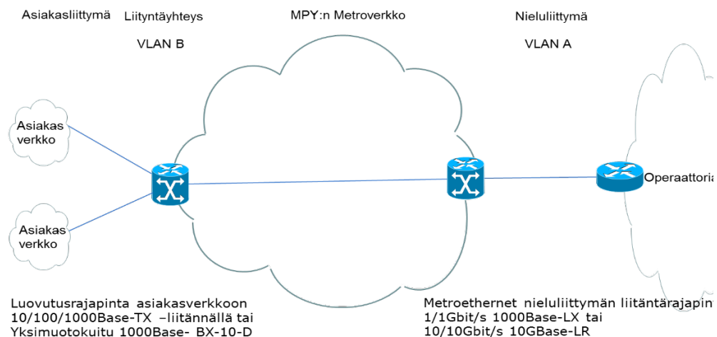
Kuva 1. Metroethernet-yhteyksien toteutus
